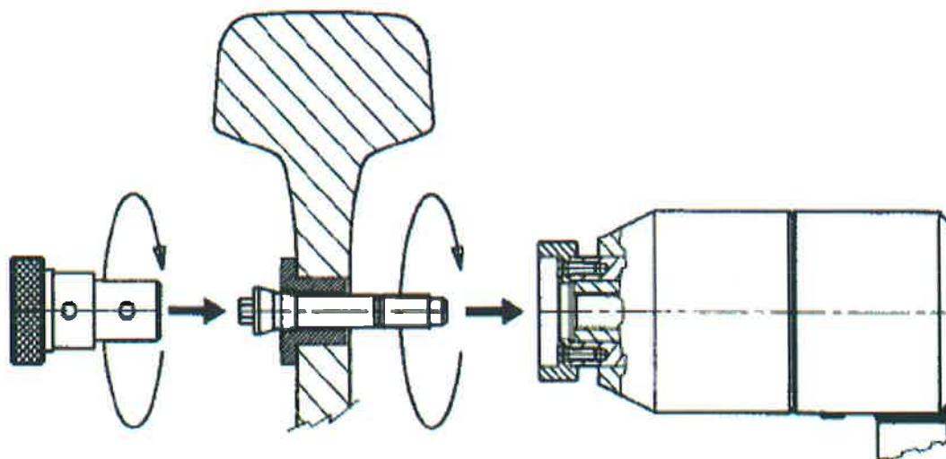
Detalj montaže tuljka za jednostruki spoj:
