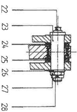
SCHNITT D - D SECTION D - D
