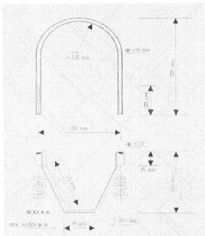
OBUJMICA ZA BETONSKI NOGAR
