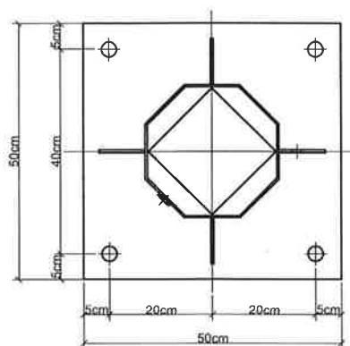
PRESJEK I - I
