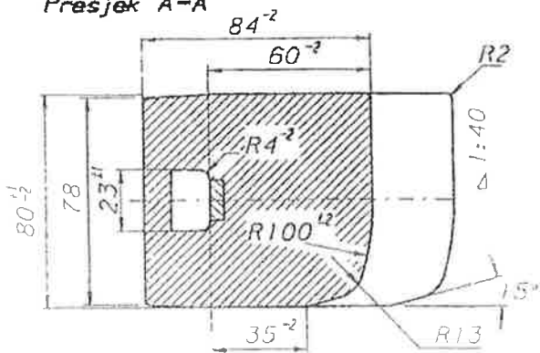
Presjek A-A
