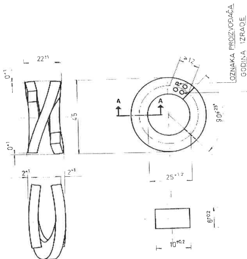
PRESJEK A-A (Mj 2:1)
