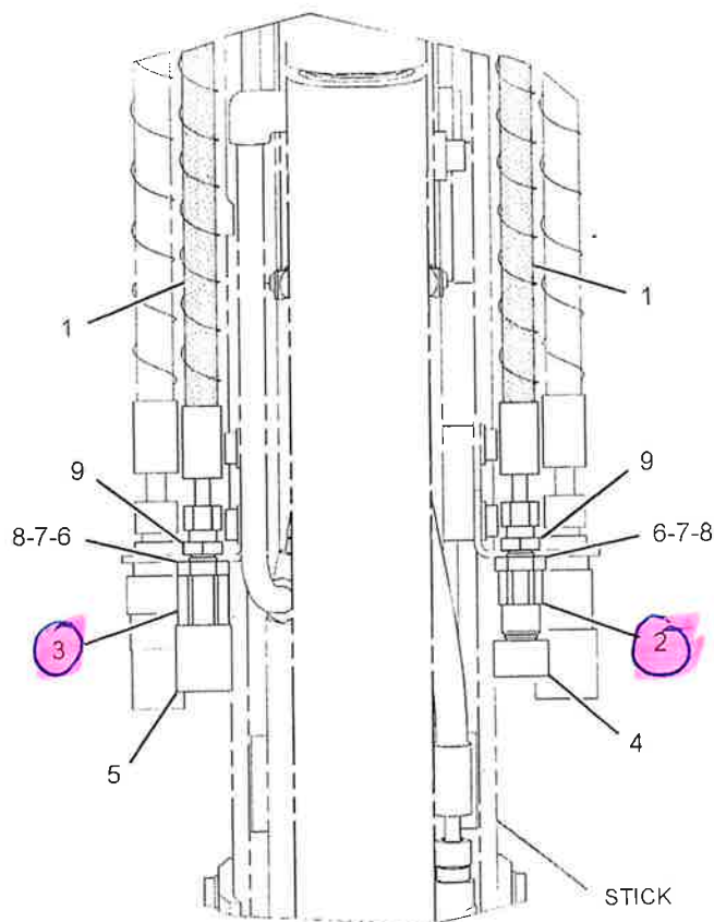
VIEW A-A
