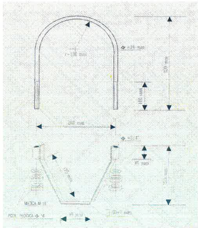
OBUJMICA ZA BETONSKI NOGAR
