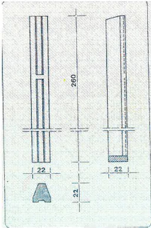
BETONSKI NOGAR
