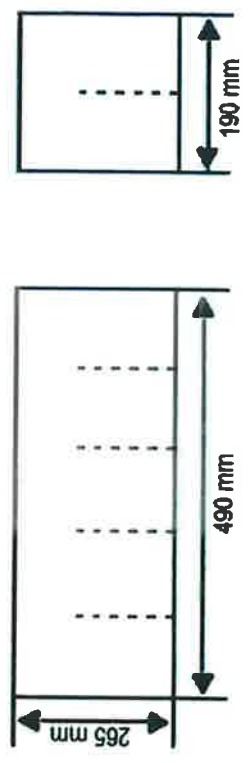
Uzdužne i poprečne pregrade od troslojne ljepenke za kartonsku kutiju tip 49
