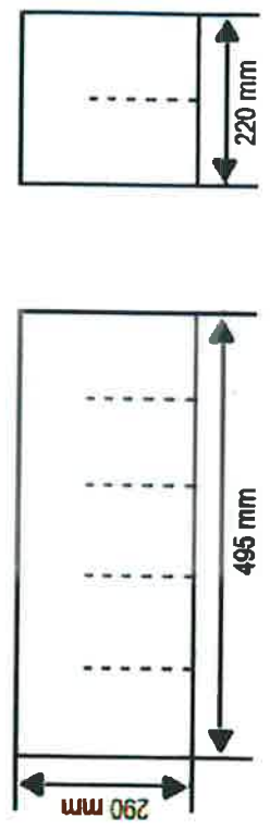
Uzdužne i poprečne pregrade od troslojne ljepenke za kartonsku kutiju tip 60
