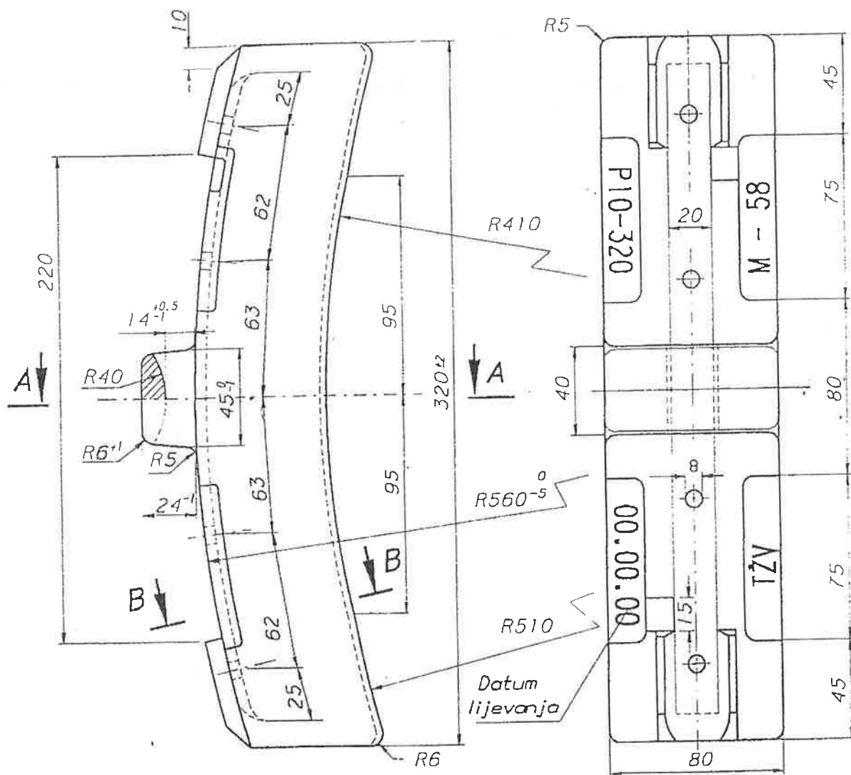
Presjek A-A
