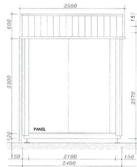
PROČELJE -C-
