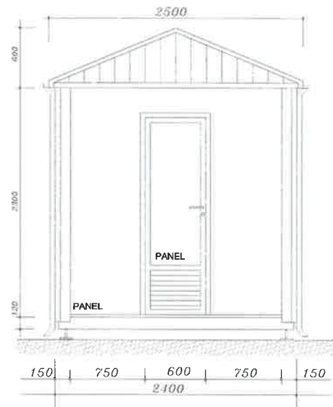
PROČELJE -A-
