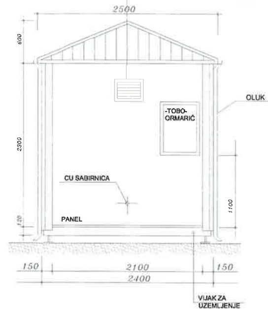
PROČELJE -D-
