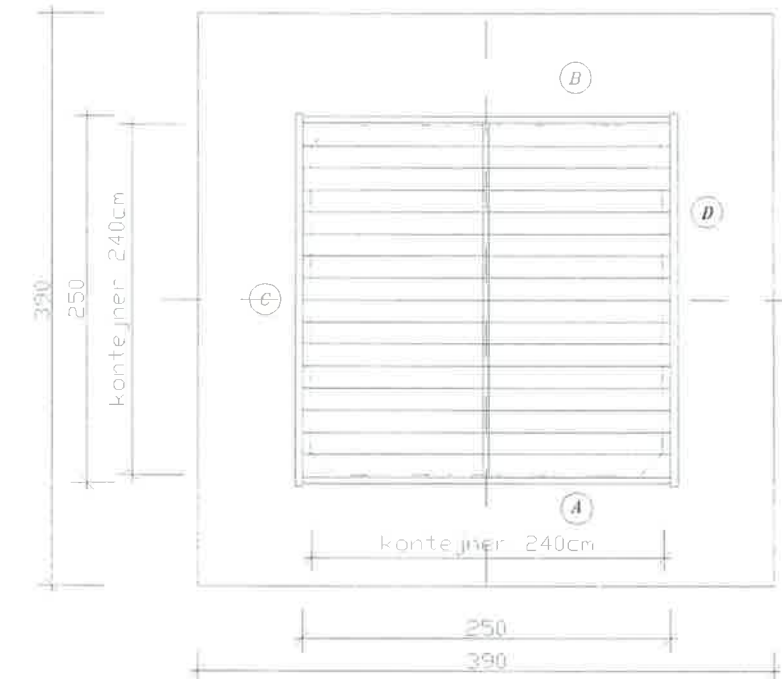
HORIZONTALNI PRESJEK KUĆICE
