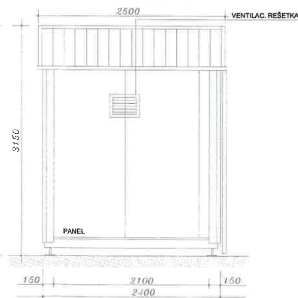
PROČELJE -D-
