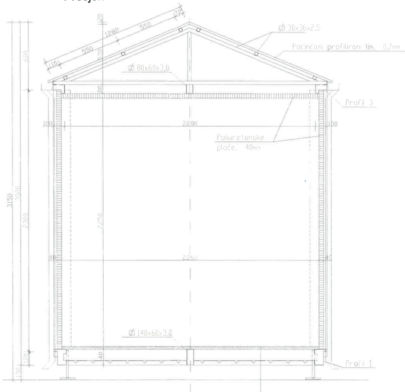
Presjek
