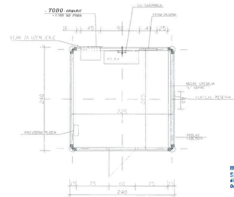
HORIZONTALNI PRESJEK KUĆICE
